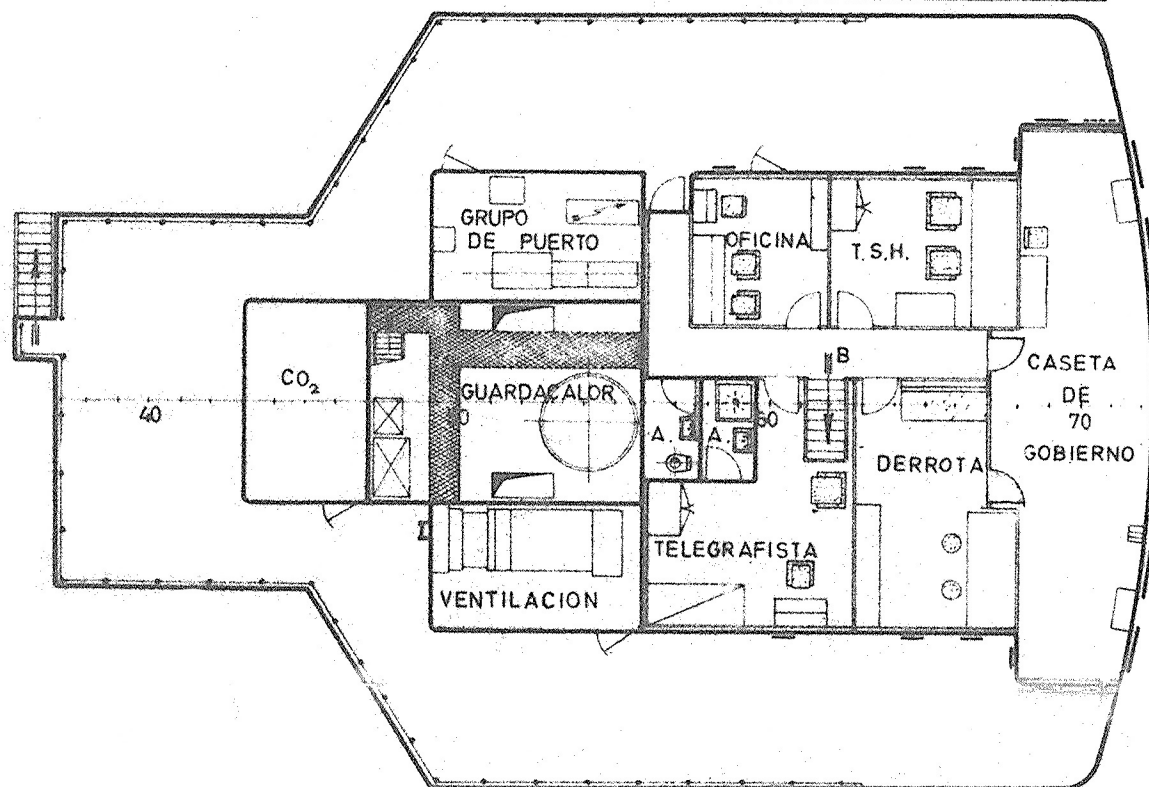
CUBIERTA PUENTE
