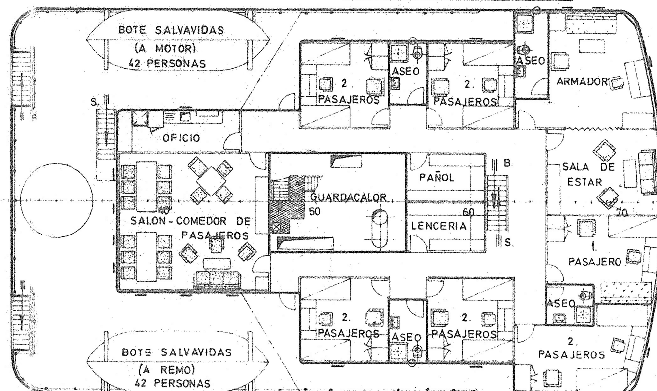
CUBIERTA BOTES
