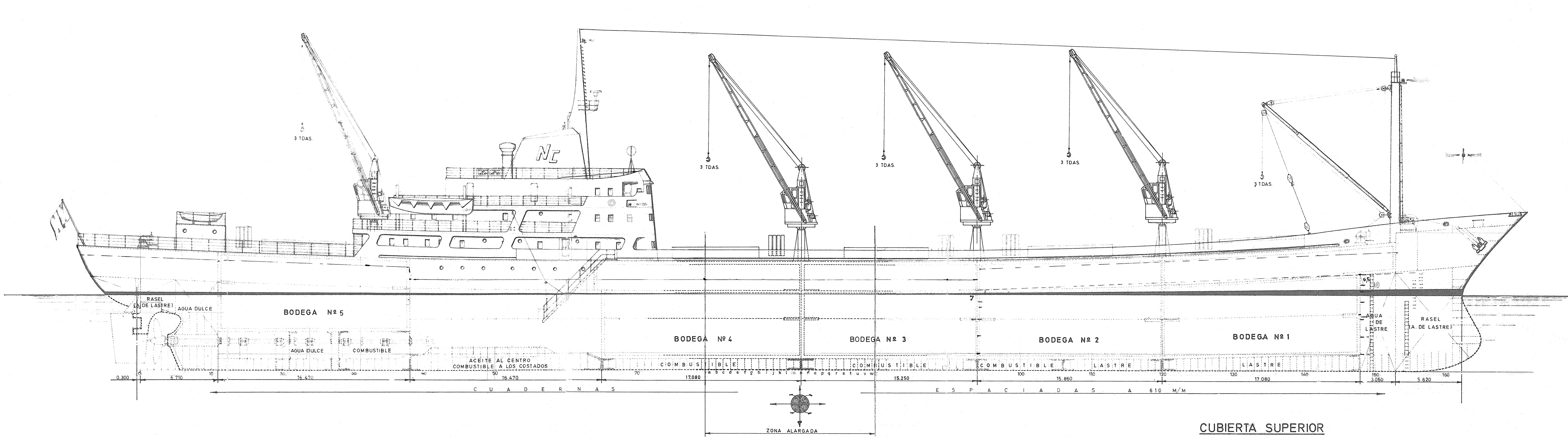
CUBIERTA SUPERIOR
