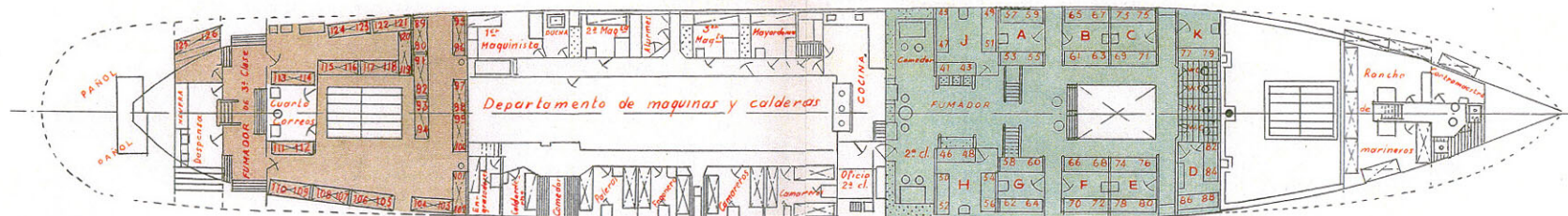
CUBIERTA PRINCIPAL
